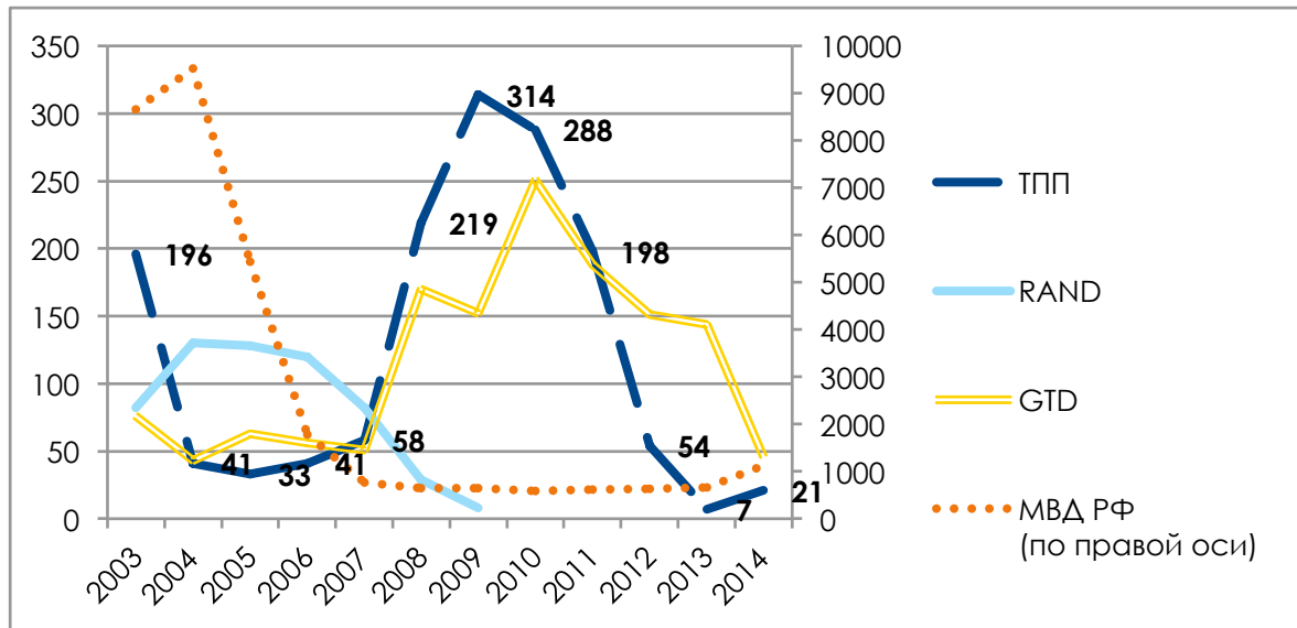
Рис. 1. Динамика численности террористических происшествий на территории России (согласно сведениям электронных баз данных)
