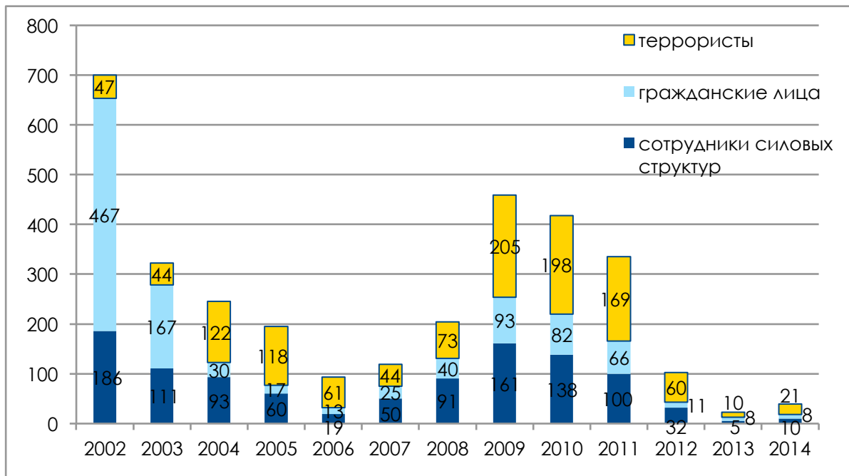
Рис. 2. Динамика численности жертв терроризма (согласно сведениям ТПП)
